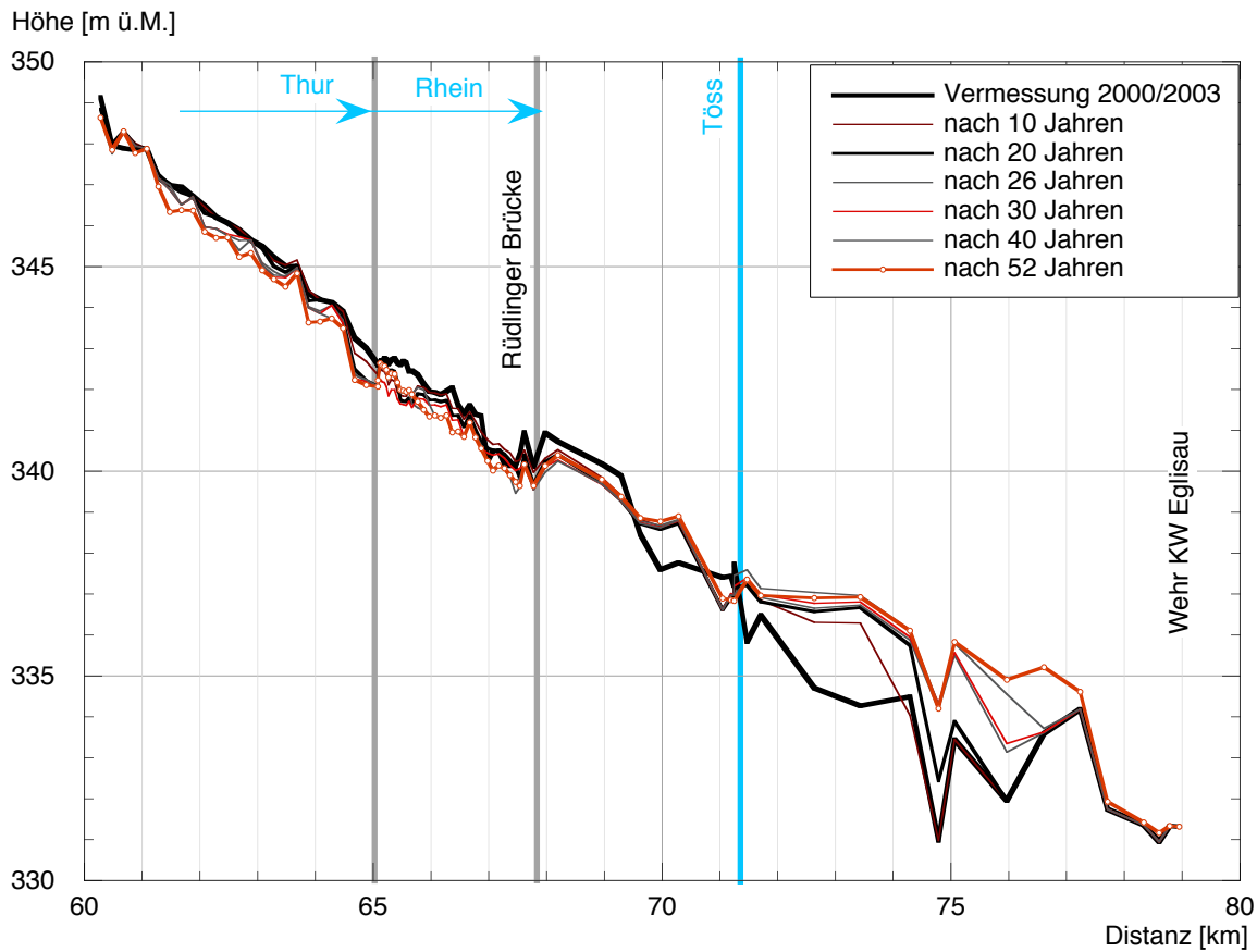
Bild 3.1 Längenprofil der mittleren Sohle im Mündungsabschnitt der Thur und der Stauhaltung Egglisau: Vermessene Sohle und berechnete Sohlenlage zu verschiedenen Zeitpunkten für den Fall mit Geschiebeeinträgen aus der Thur von 13'000 m 3 /Jahr und aus der Töss von 3'000 m 3 /Jahr.
