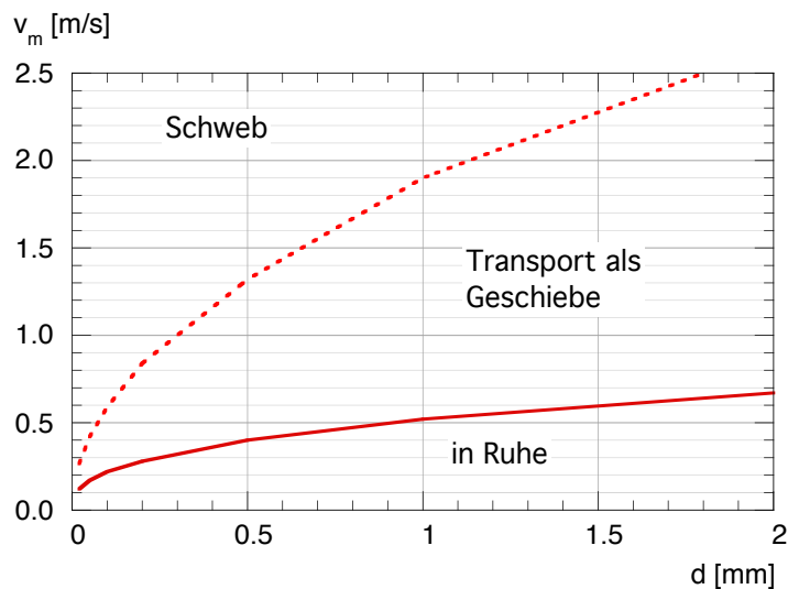
Bild 2.1 Abhängigkeit des Transportverhaltens von Schwebstoffkörnern mit unterschiedlichem Durchmesser d von der mittleren Fließgeschwindigkeit v_m .
